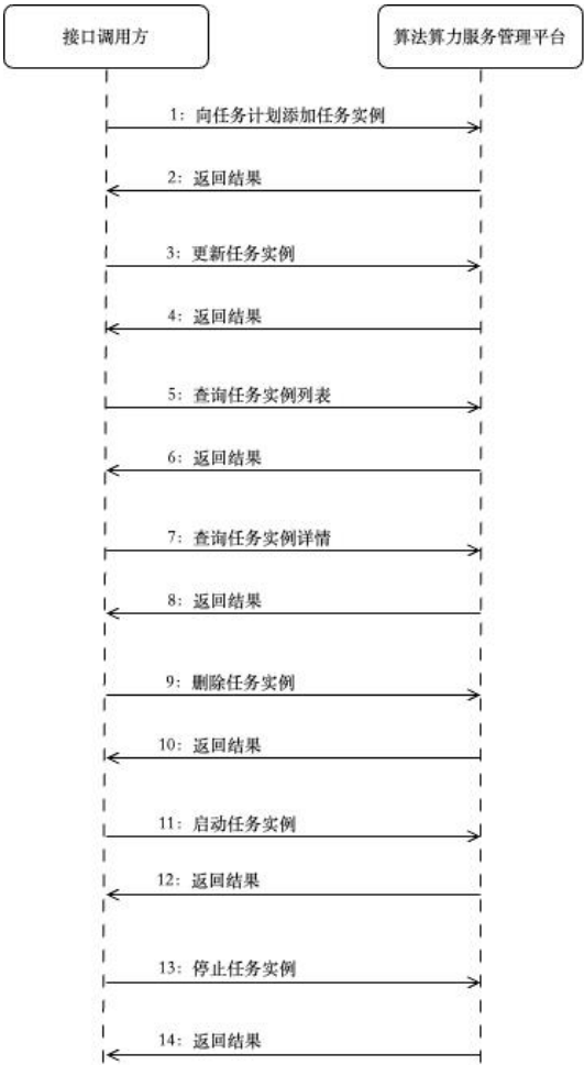
图 9 任务实例接口调用流程
