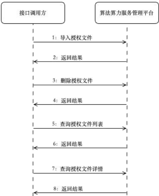
图 11 离线鉴权接口调用流程
