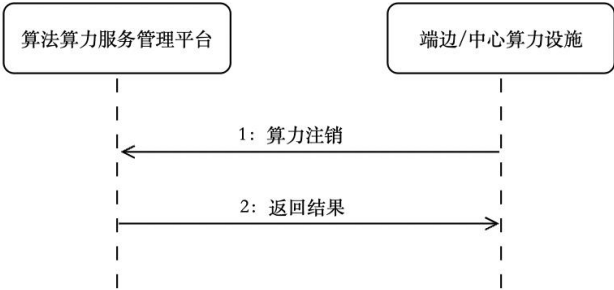
图 13 算力注销接口流程
