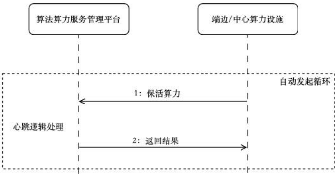
图 14 算力保活接口流程
