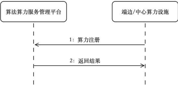
图 12 算力注册接口流程
