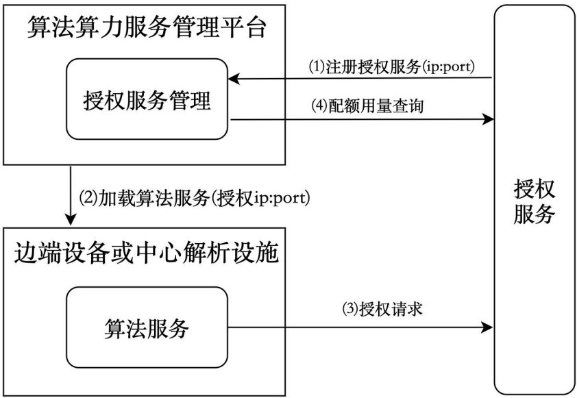
图 3 在线鉴权流程示意图
