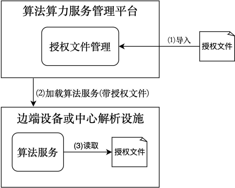
图 4 离线鉴权流程示意图
