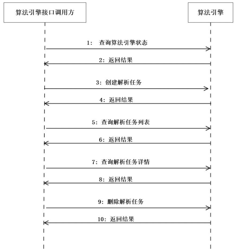
图 2 算法引擎接口调用流程
